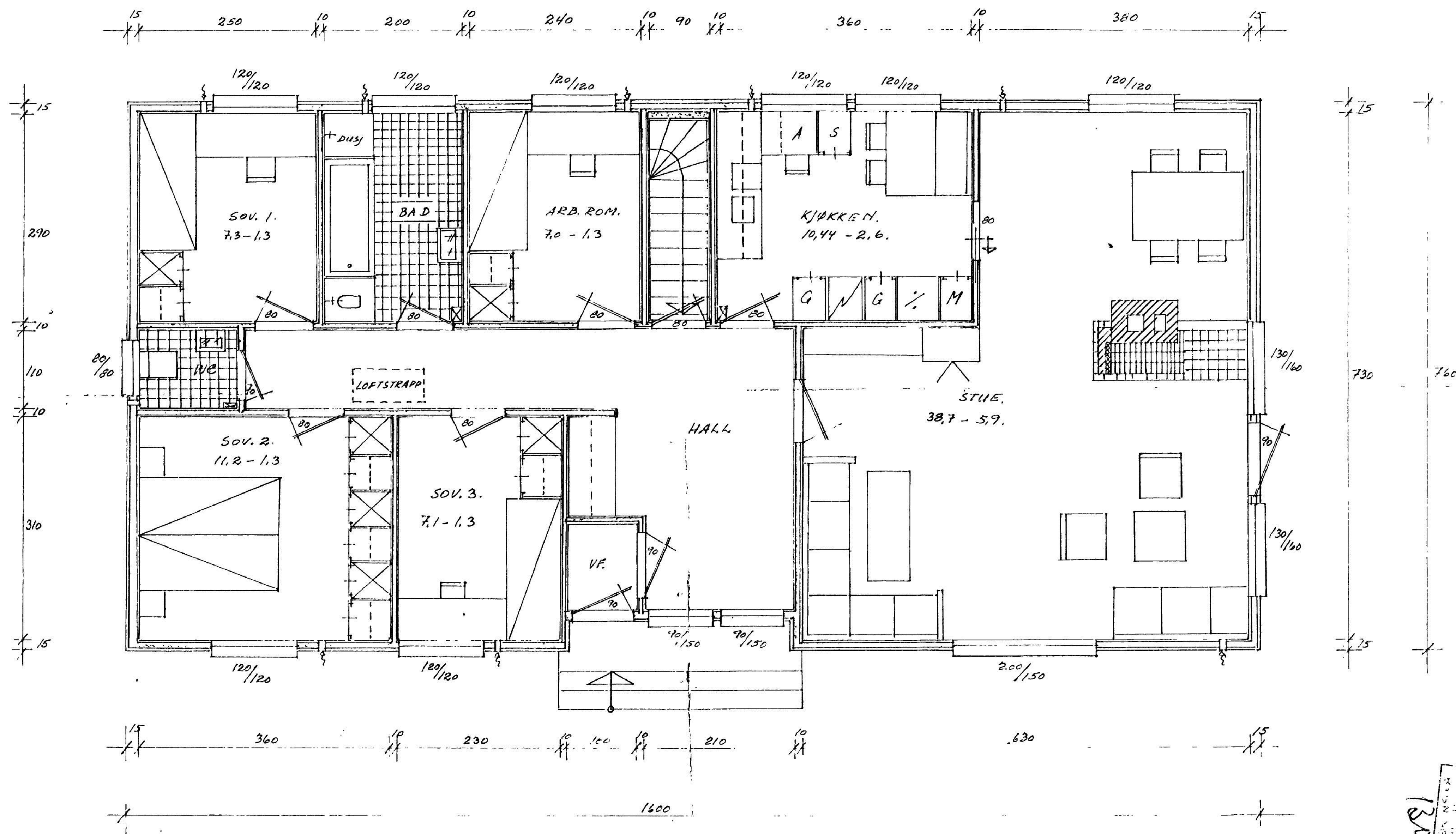
PLAN 1. ETASJE.
